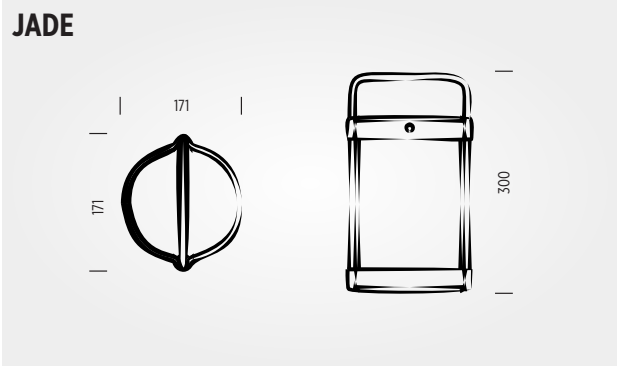
LxPxA: ø171x300mm
