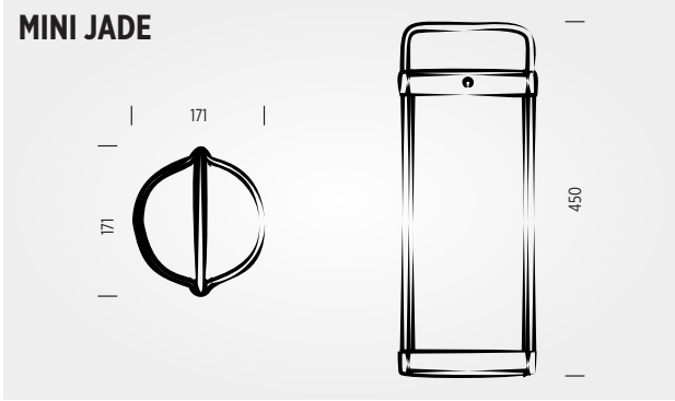
LxPxA: ø171x450mm
